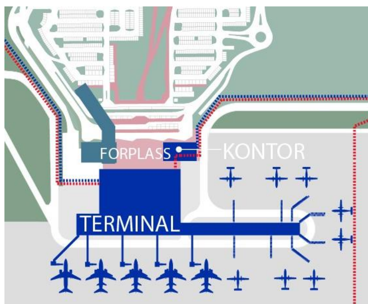
Figur 9: Situasjonsplan av terminalkomplekset med plassering av terminal, kontorfløy, forplasset med underliggende parkeringsarealer og varemottak/økonomigård, samt mulig hotell
