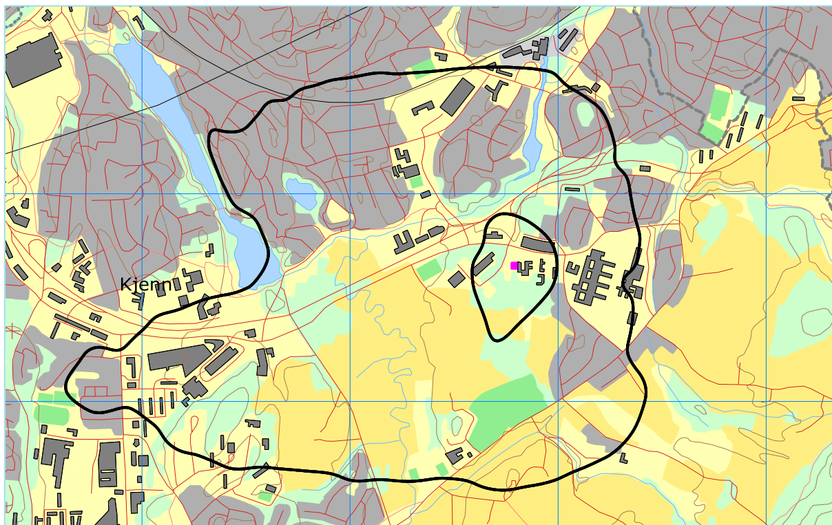
Figur 9-3 L_{den} 52 og 62 dBA for prognosesituasjonen. M 1:25 000.
