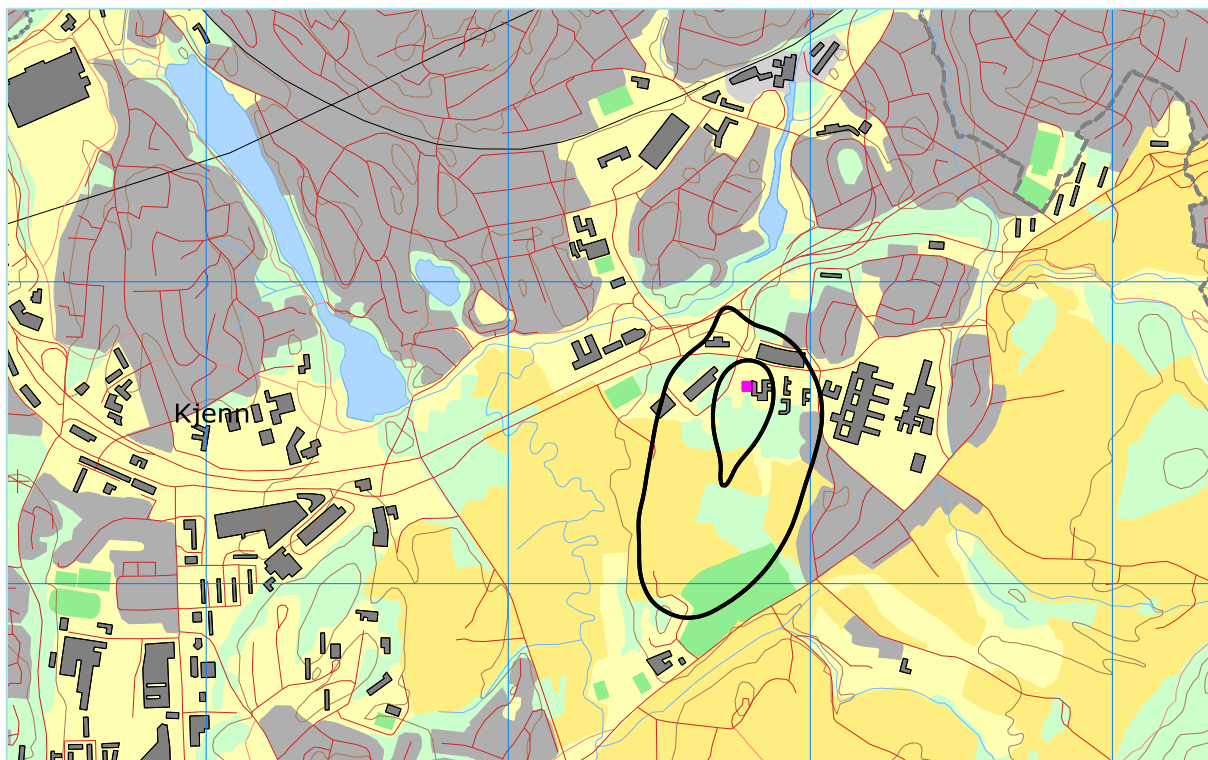
Figur 9-2 L_{sas} 80 og 90 dBA for dagens situasjon. M 1:25 000.
